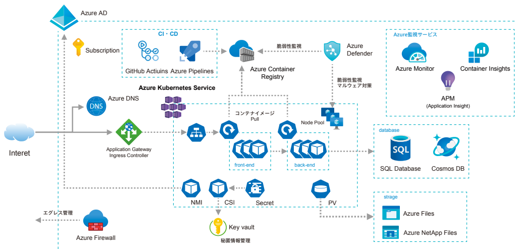
Azure Kubernetes Service(AKS)を利用したコンテナアプリケーションの構成例
