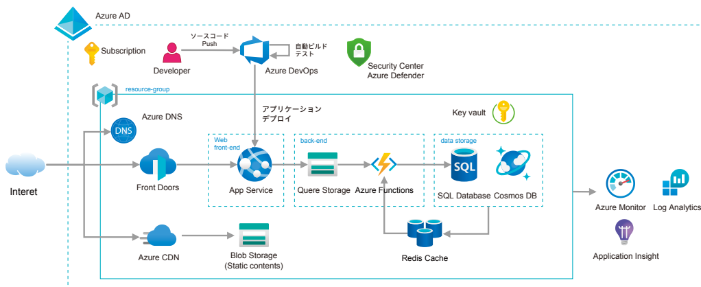
スケーラブルなWebサービスの構成例
