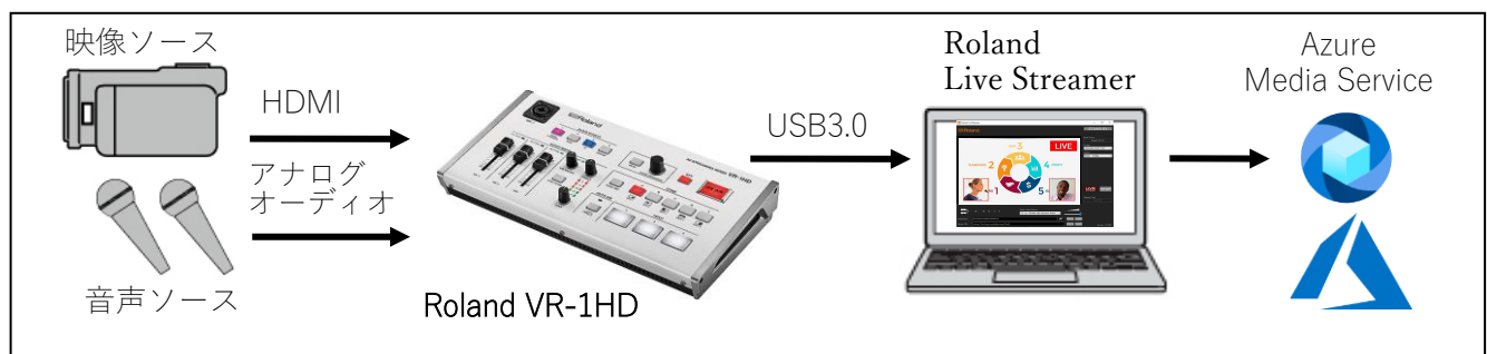
図 2 ライブ配信システム例 (スイッチャー: Roland VR シリーズ)
